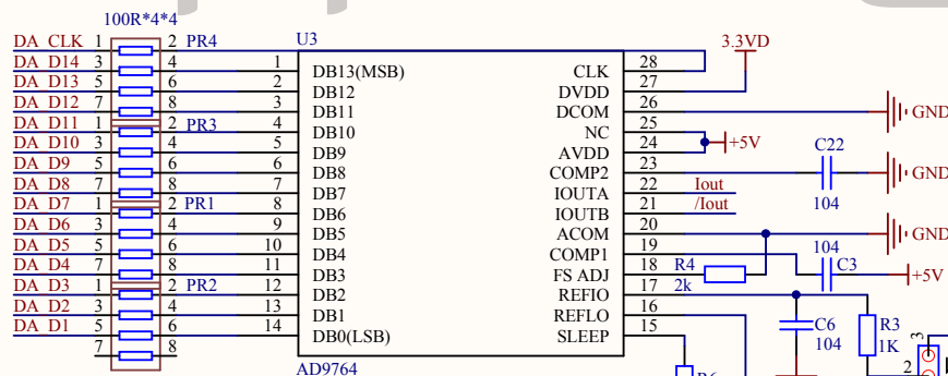
AD9764模块
